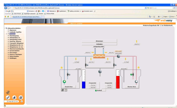
Figuur 2 Bronregeling
